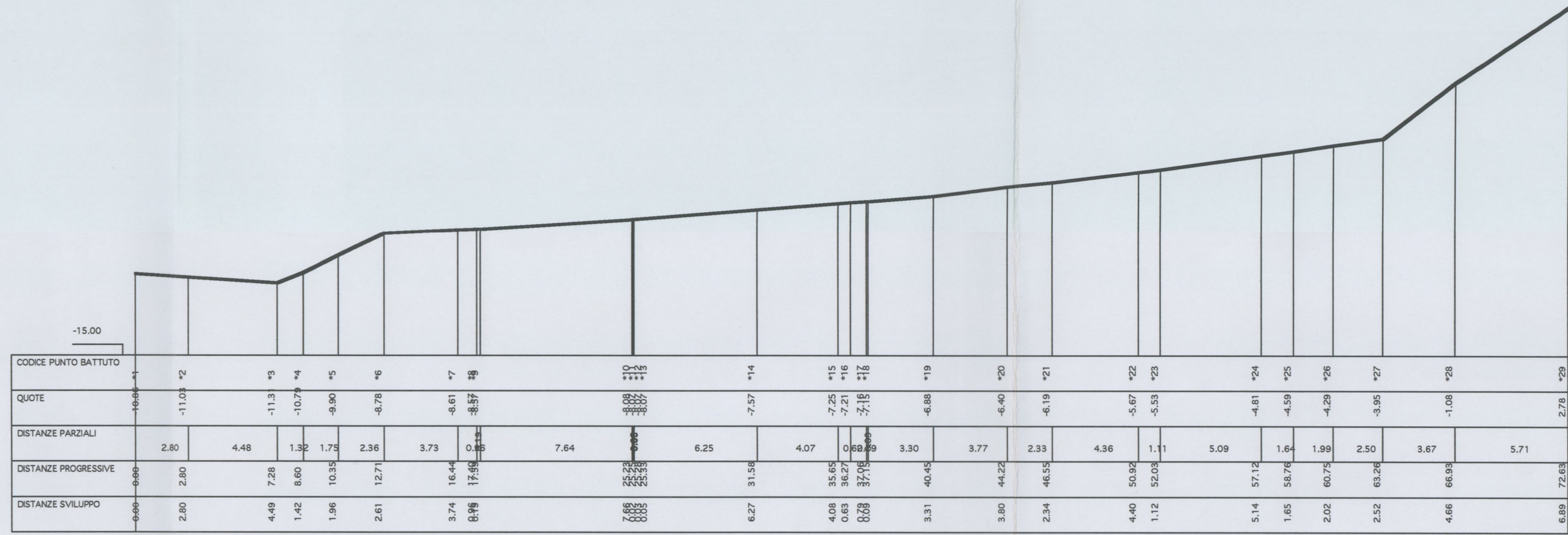
Sezione: 4 Scala H 1:200 Scala V 1:200 SEZIONE AMBIENTALE 4 - 4 , scala 1:200
