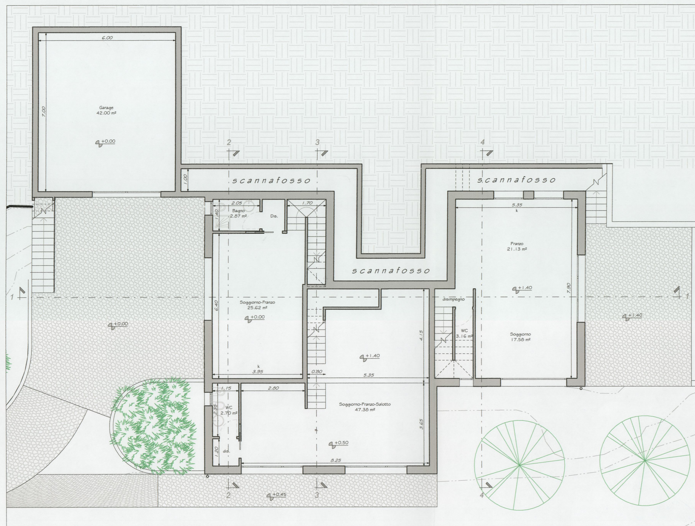
○ Pianta Piani Inferiori
