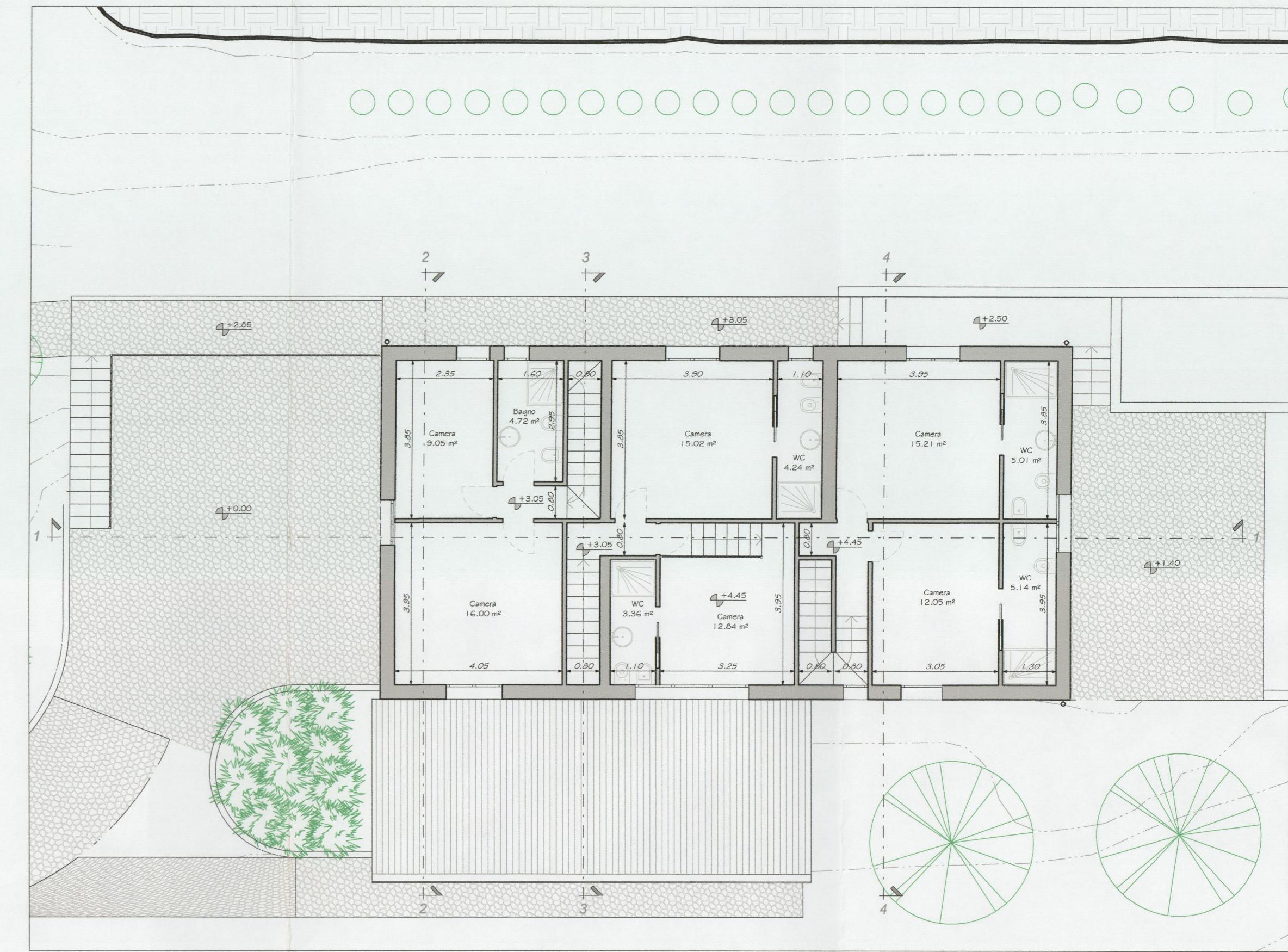
○ Pianta Piani Superiori
