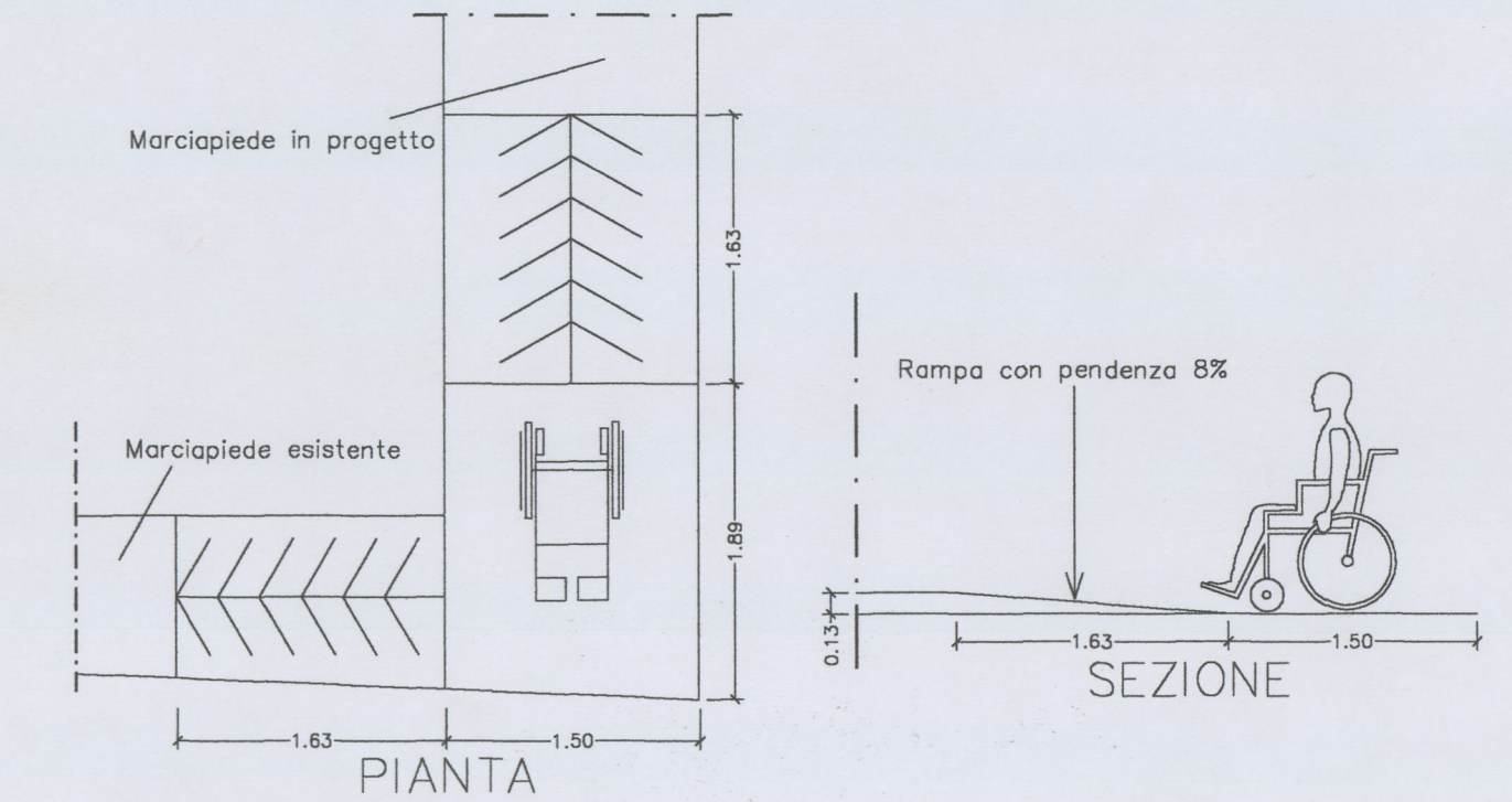
PARTICOLARE ACCESSO AI MARCIAPIEDI SCALA 1:50
