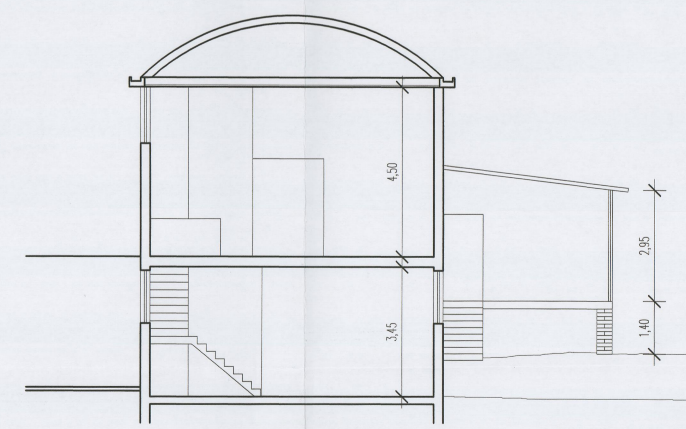
SEZIONE B-B
