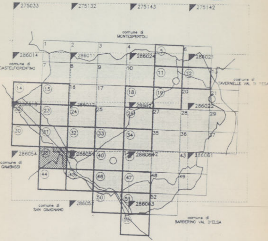
TAV. N°2 DESTINAZIONI D'USO E ORIENTAMENTI PER IL RIassetto DEI CENTRI URBANI 1/2.000
