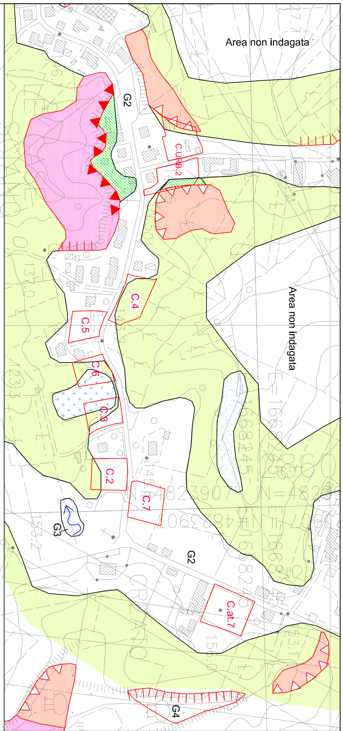
TAV. 2 - SCIANO Carta geomorfologica scala 1/3000
